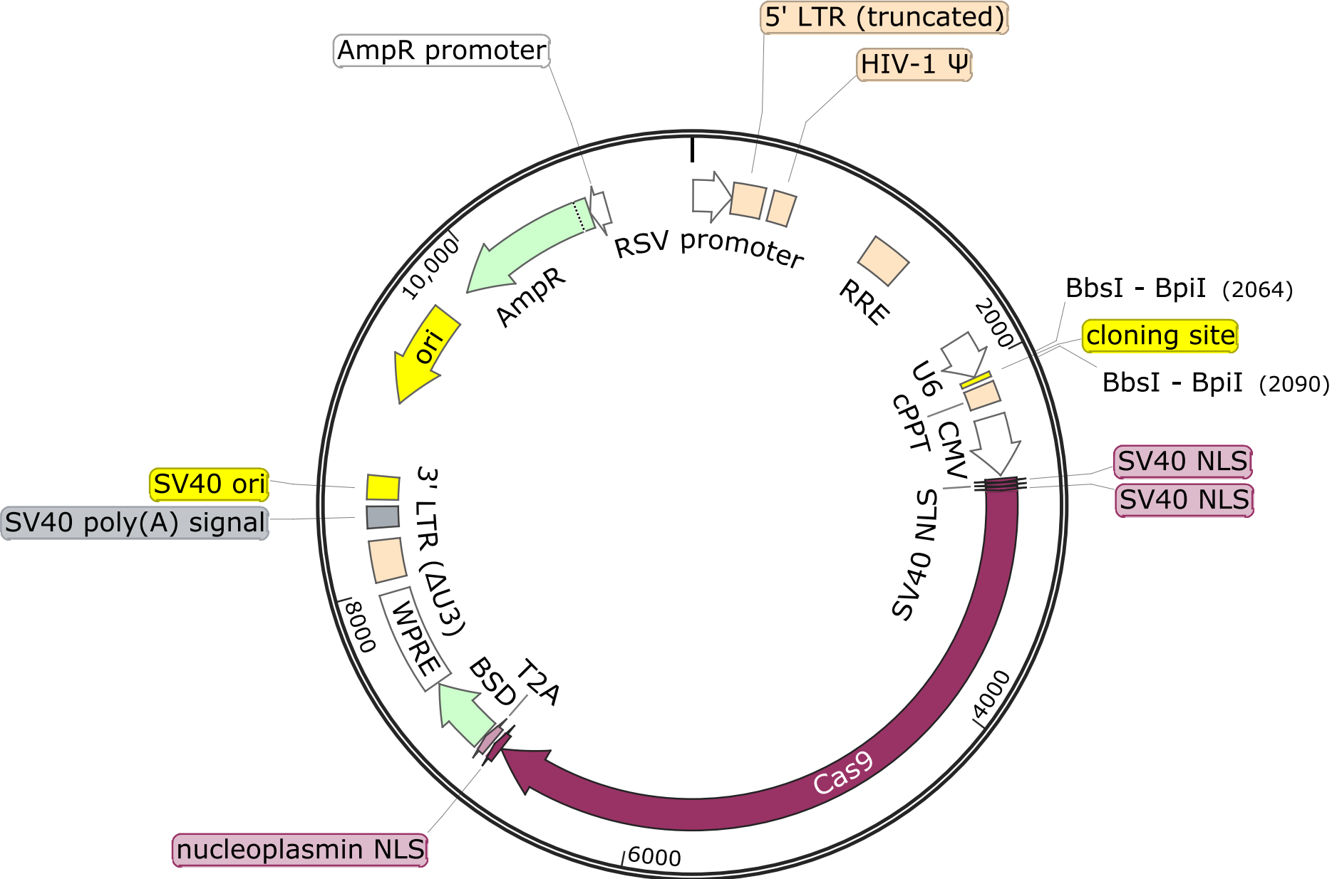
Collecta-pRSGCCB-U6-sg-HTS6C-CMV-Cas9-2A-Blast
