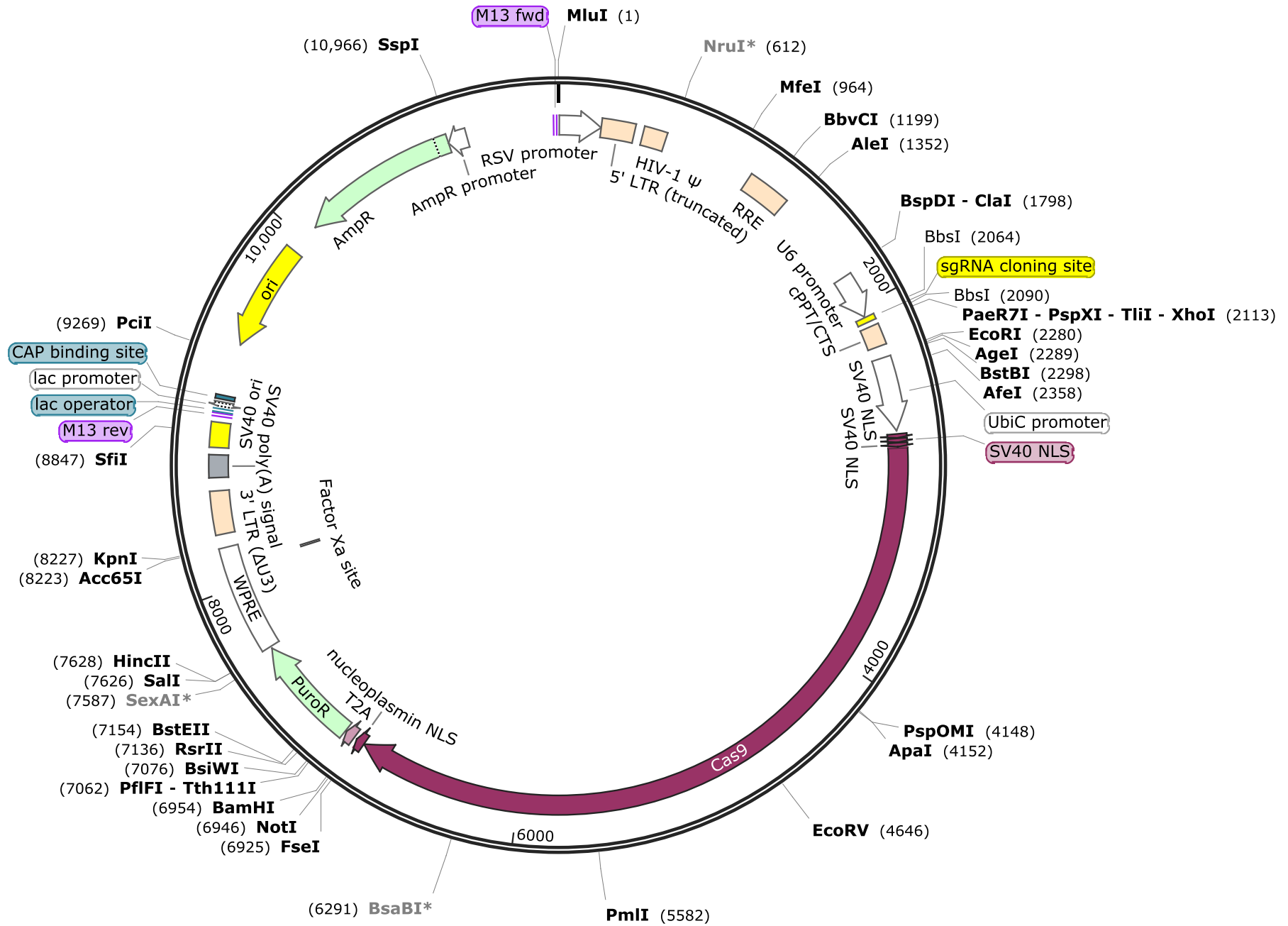
Collecta-pRSGCUP-U6-sg-HTS6C-UbiC-Cas9-2A-Puro 11,553 bp
